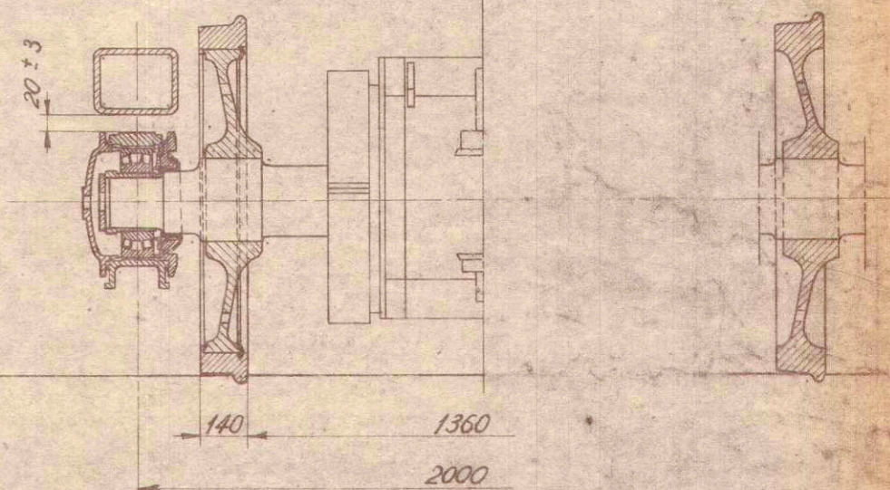
1/2 Coupe. B B. 1/2 Doorsnede
