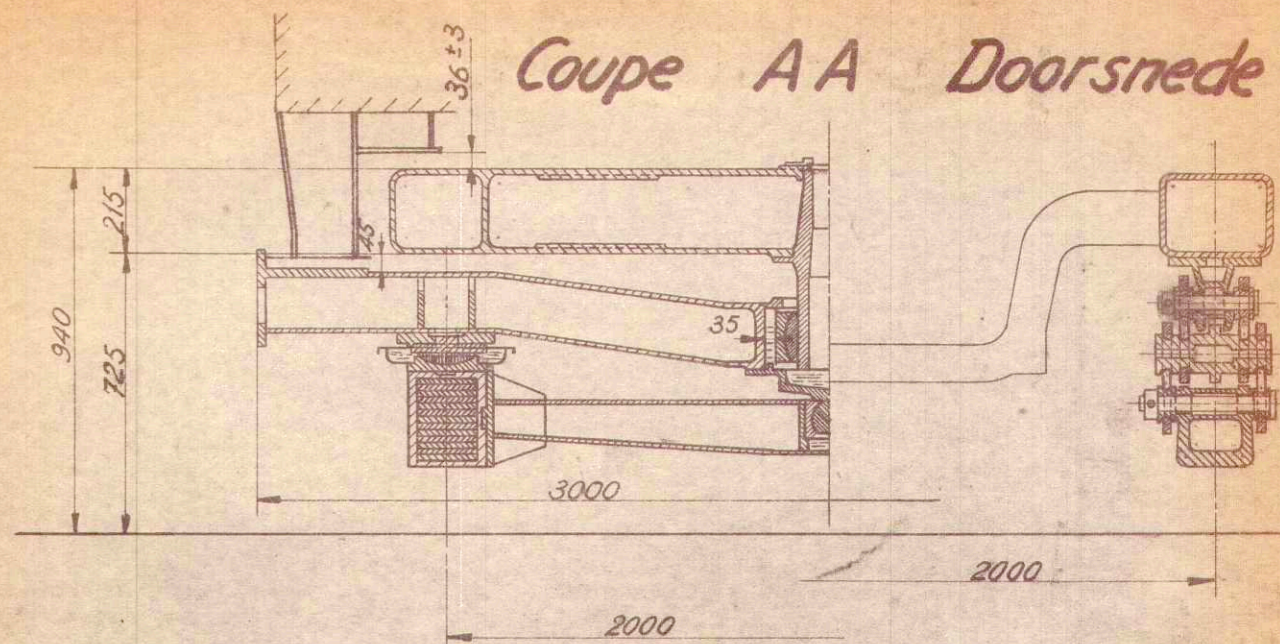
Coupe A A Doorsnede
