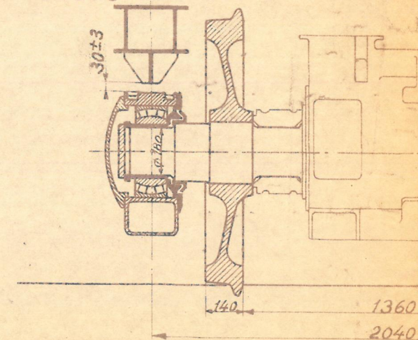
1/2 coupe doorsnede CC.
