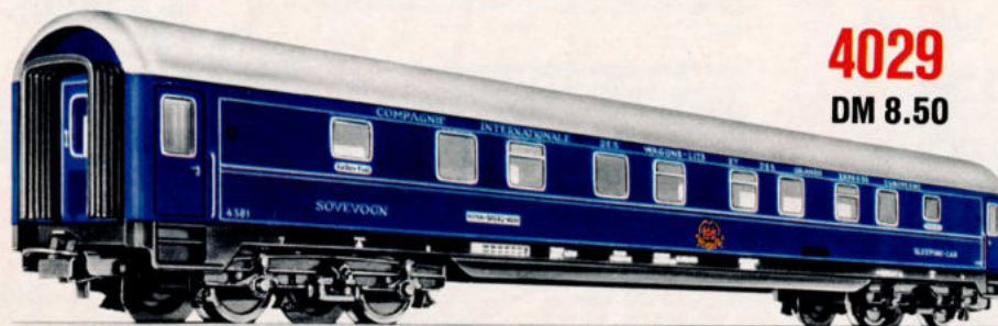
4029 D-Zug-Schlafwagen · Modell der Internationalen Schlafwagengesellschaft (ISG Nr. 4581) · 4-achsig · Abnehmbares Dach · Eingesetzte Fenster mit plastischen Rahmen · Blau · Dach silbern, grau getönt · Vorbildgetreue Beschriftung · Faltenbalgimitationen an den Stirnseiten · Länge 24 cm
