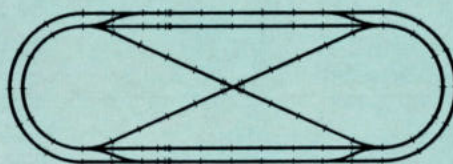
Zweigleisiges Oval mit doppelter Kehrschleife
