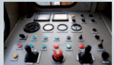
Poste de conduite ergonomique avec commande traction/freinage par joystick
