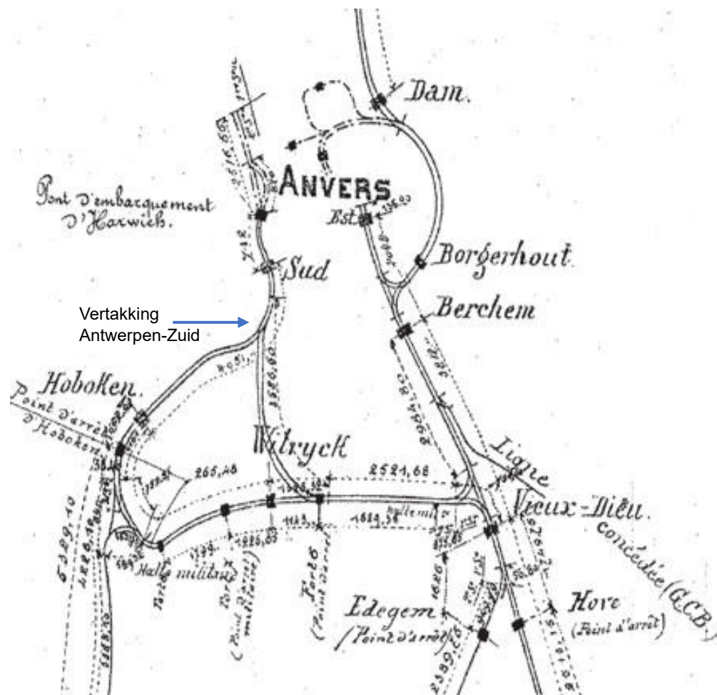
De spoorlijnen ten zuiden van Antwerpen in 1896. Het lijngedeelte tussen Antwerpen-Zuid – d.w.z. tussen de vertakking Antwerpen-Zuid en de fortenlijn in Wilrijk – had een lengte van slechts 3,368 km en kwam in dienst in 1894.
