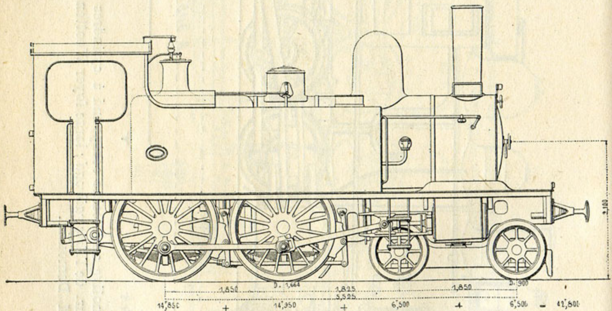
Fig. 280. — Locomotive-tender à 2 essieux couplés et à bogie, avec cylindres extérieurs, du chemin de fer du Nord. D'après M. Demoulin.
